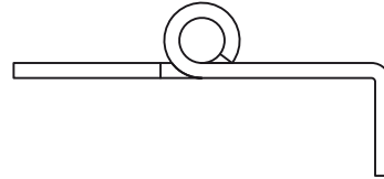
Abwicklung und Profilierung einer oder beider Scharnierhälften
